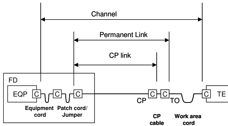
Abbildung 1: 4-Connector Channel (Übertragungsstrecke) nach ISO/IEC 11801: 2002
