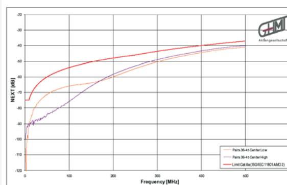
Beispiel 1: Ergebnisse aus NEXT Messungen der Paar-kombination 3,6 / 4,5 (Center Low und High)
