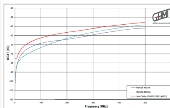
Beispiel 2: Ergebnisse aus NEXT Messungen der Paar-kombination 3,6 / 4,5 (Low und High)
