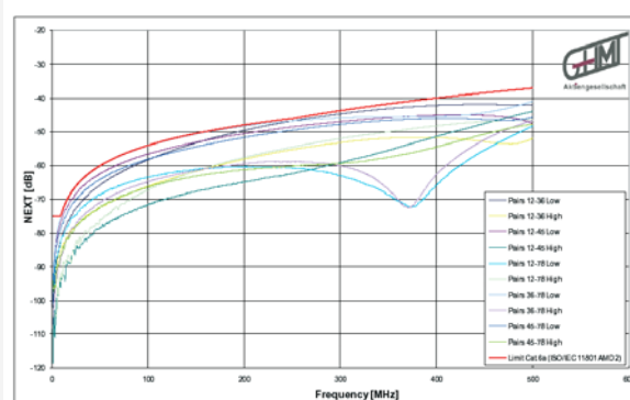
Beispiel 3: Ergebnisse aus NEXT Messungen der restlichen Paarkombinationen
