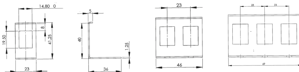
Montagewinkel 501343, 501344 und 501345 (Maßangaben ohne Befestigungsclips)
